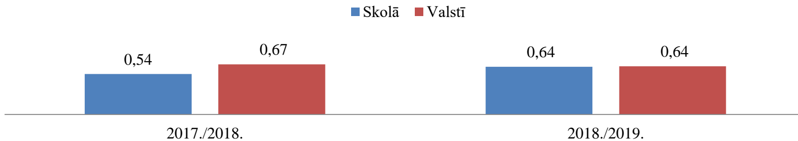
2.6. attēls. Sasniegumu vidējie rādītāji 9.klasē VPD –latviešu valodā
