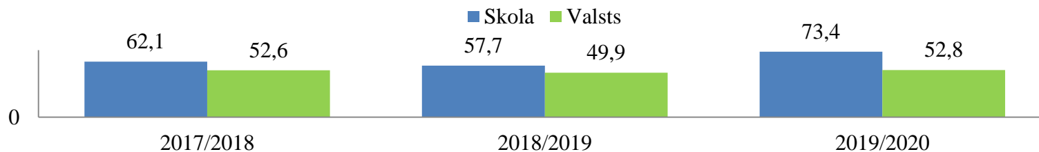
2.11. attēls. Sasniegumu vidējie rādītāji latviešu valodas CE kopvērtējumā (%) skolā un valstī
