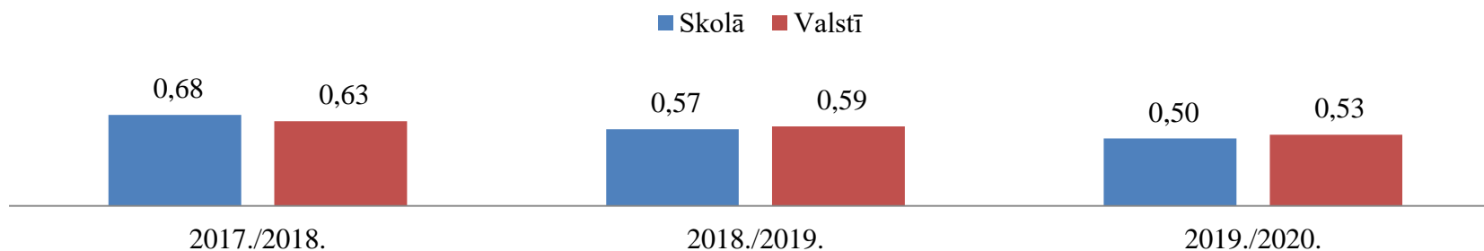
2.5. attēls. Sasniegumu vidējie rādītāji 6.klasē VPD –dabaszinībās
