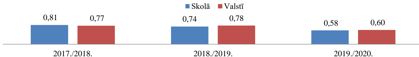
2.2. attēls. Sasniegumu vidējie rādītāji 3.klasē VPD – matemātikā
