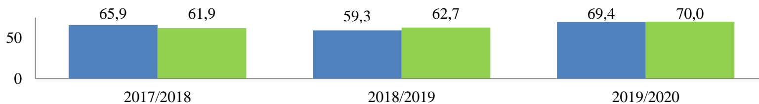
2.12. attēls. Sasniegumu vidējie rādītāji angļu valodas CE kopvērtējumā (%) skolā un valstī
