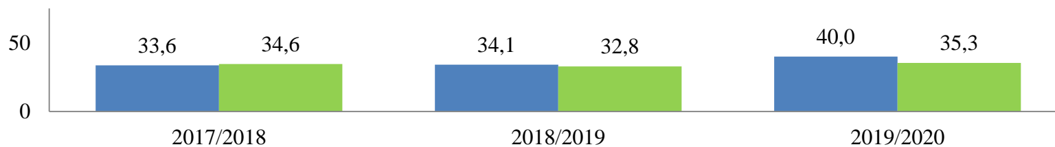
2.13. attēls. Sasniegumu vidējie rādītāji krievu valodas CE kopvērtējumā (%) skolā un valstī
