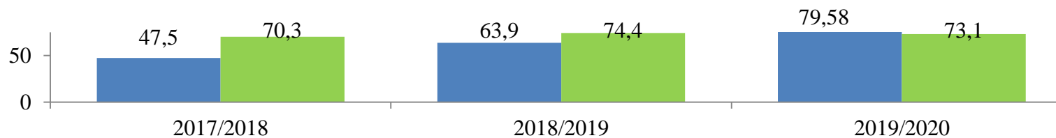
2.12. attēls. Sasniegumu vidējie rādītāji angļu valodas CE kopvērtējumā (%) skolā un valstī
