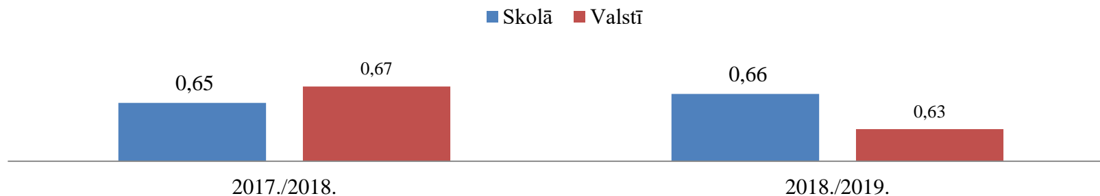
2.10. attēls. Sasniegumu vidējie rādītāji 9.klasē VPD –Latvijas vēsturē
