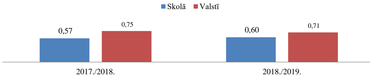
2.8. attēls. Sasniegumu vidējie rādītāji 9.klasē VPD –krievu valodā
