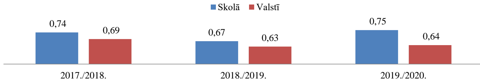
2.3. attēls. Sasniegumu vidējie rādītāji 6.klasē VPD – latviešu valodā
