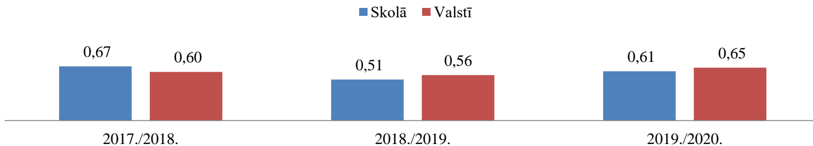
2.4. attēls. Sasniegumu vidējie rādītāji 6.klasē VPD – matemātikā
