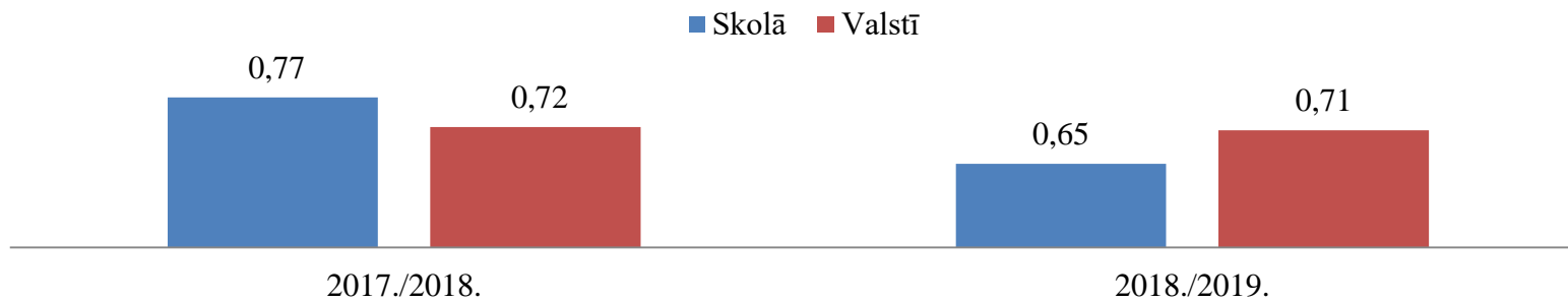
2.7. attēls. Sasniegumu vidējie rādītāji 9.klasē VPD –angļu valodā
