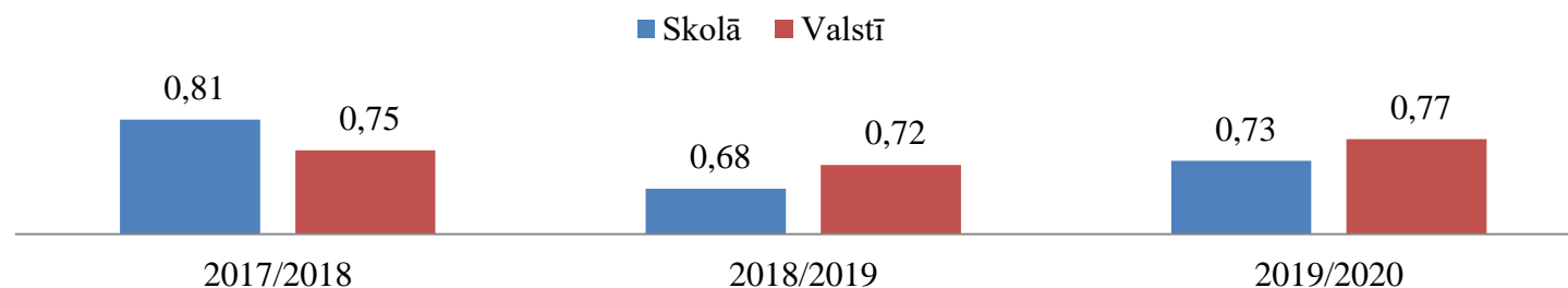
2.1. attēls. Sasniegumu vidējie rādītāji 3.klasē VPD – latviešu valodā
